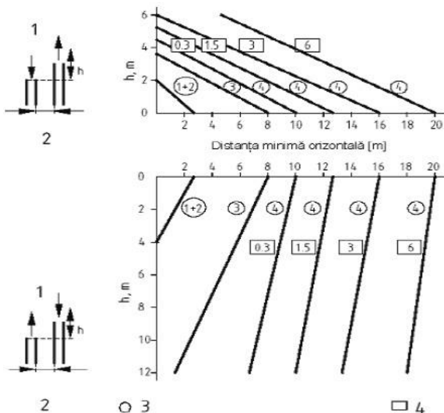
Figura 6.6.2. - Distanțe minime între gura de evacuare și cea de introducere a aerului
