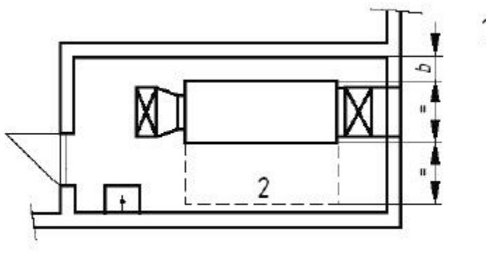
Figura 6.6.1. - Dispunerea instalațiilor de tratare a aerului (vedere în plan)
