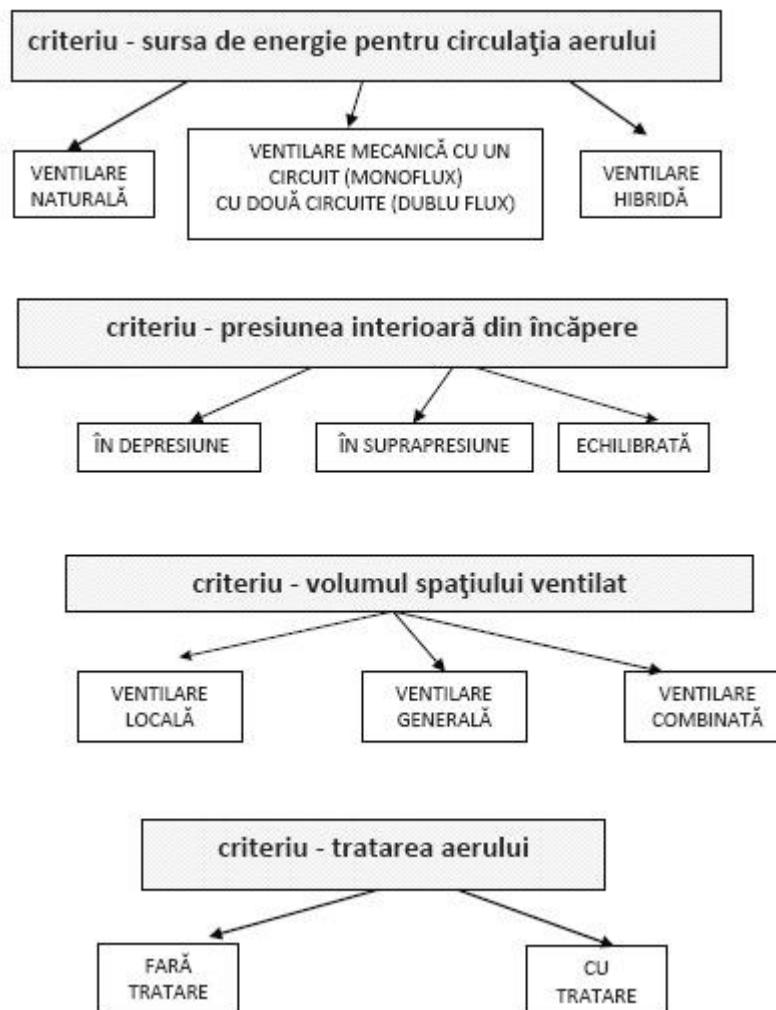
Figura 3.1. Clasificarea instalațiilor de ventilare
