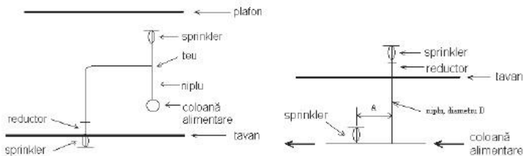
Figura 7.4. Amplasarea sprinklerelor în spațiul dintre nivelul tavanelor și a acoperișurilor
