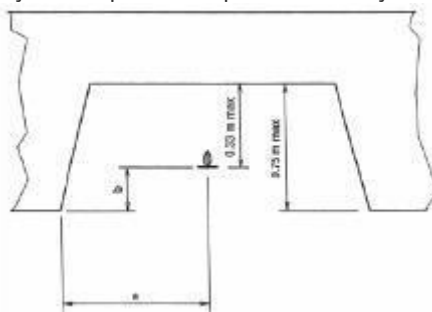
Figura 7.14 - Distanțe de amplasare a sprinklerelor față de marginea inferioară a unui plafon ondulat
