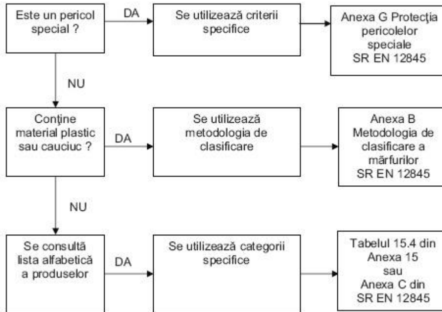
Figura 7.2. Schemă de determinare a claselor de pericol la incendiu pentru depozite (conform SR EN 12845)
