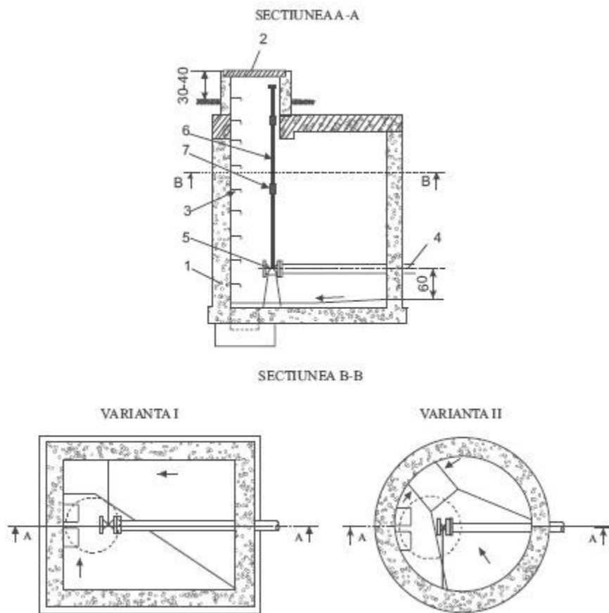
Figura. 12.2 Cămin de alimentare directă cu apă a pompelor mobile de tip B
