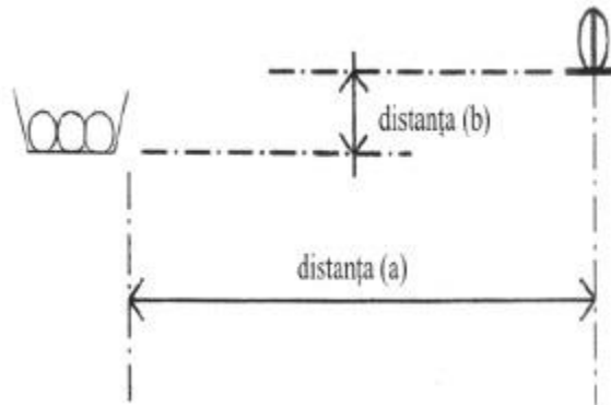
Figura 7.17 - Nomogramă de stabilire a distanțelor de amplasare a sprinklerelor față de elementele vecine
